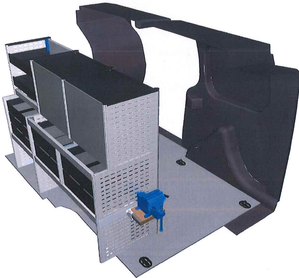
Rys. 3 Lewa ścianka z zabudową. Widok od tyłu.
