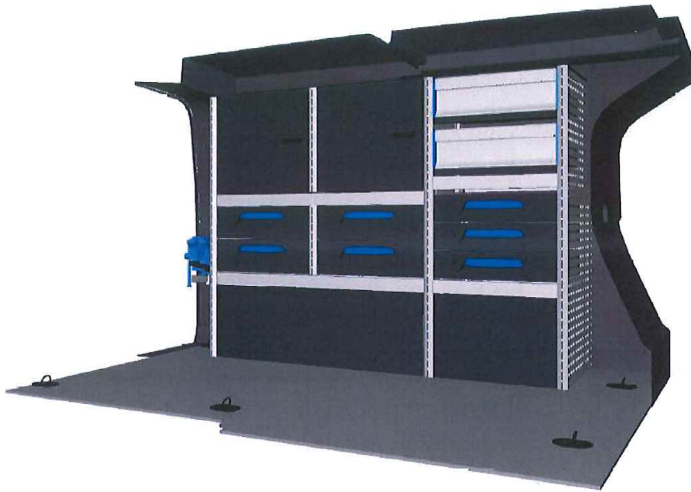
Rys. 2 Lewa ścianka z zabudową. Widok od frontu.
