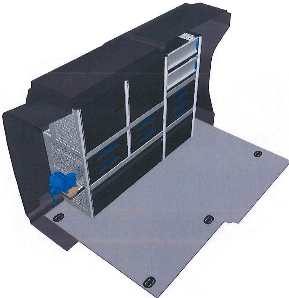
Rys. 1 Lewa ścianka z zabudową
