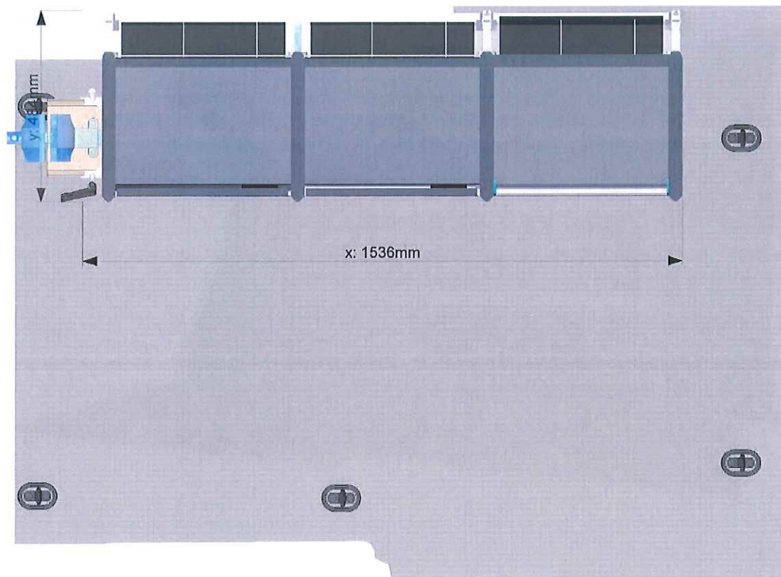
Rys. 6 Zabudowa . Widok z góry.
