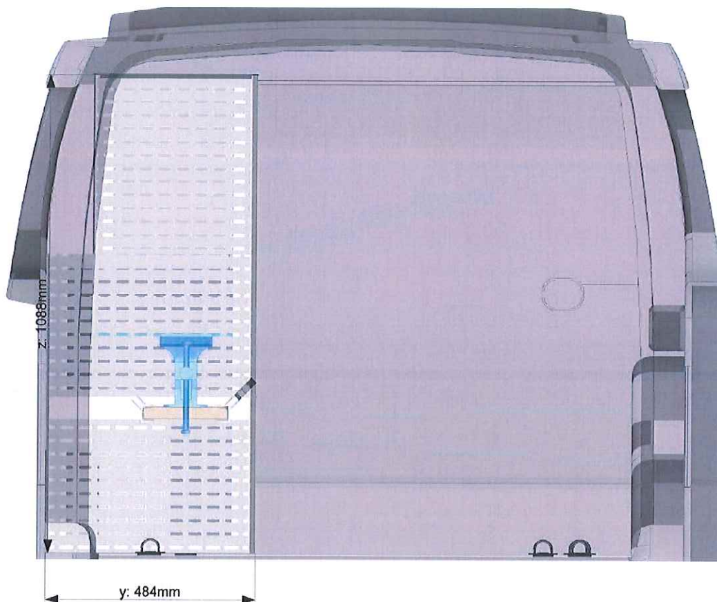
Rys. 8 Widok na zabudowę od strony tylnych drzwi.
